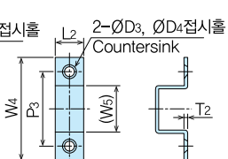
브라켓A BracketA (SDA-30-1)
