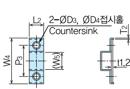
브라켓A BracketA (SDA-30-2)
