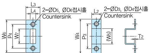
브라켓B BracketB
